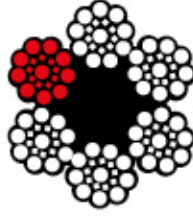
6x19 Seale
