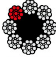
8x19 Seale
